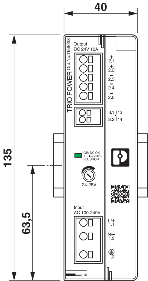
Rysunek wymiarowy
