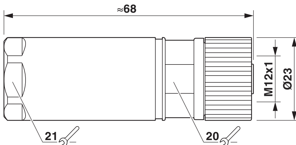
Rysunek wymiarowy
