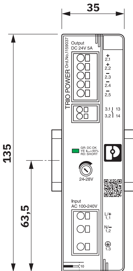
Rysunek wymiarowy
