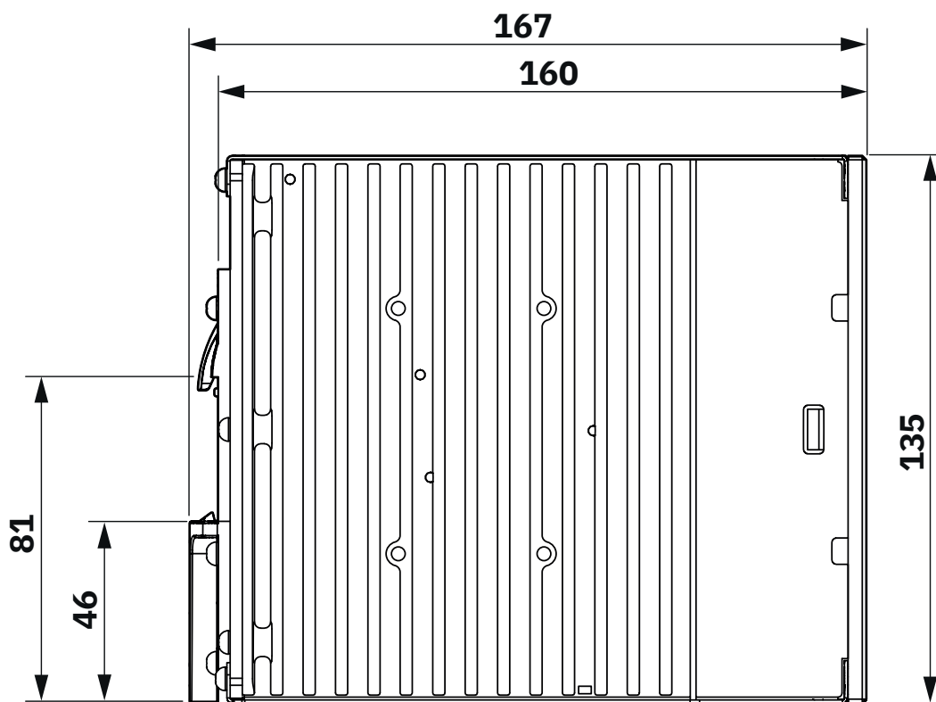
Wymiary urządzenia (wymiary w mm)
