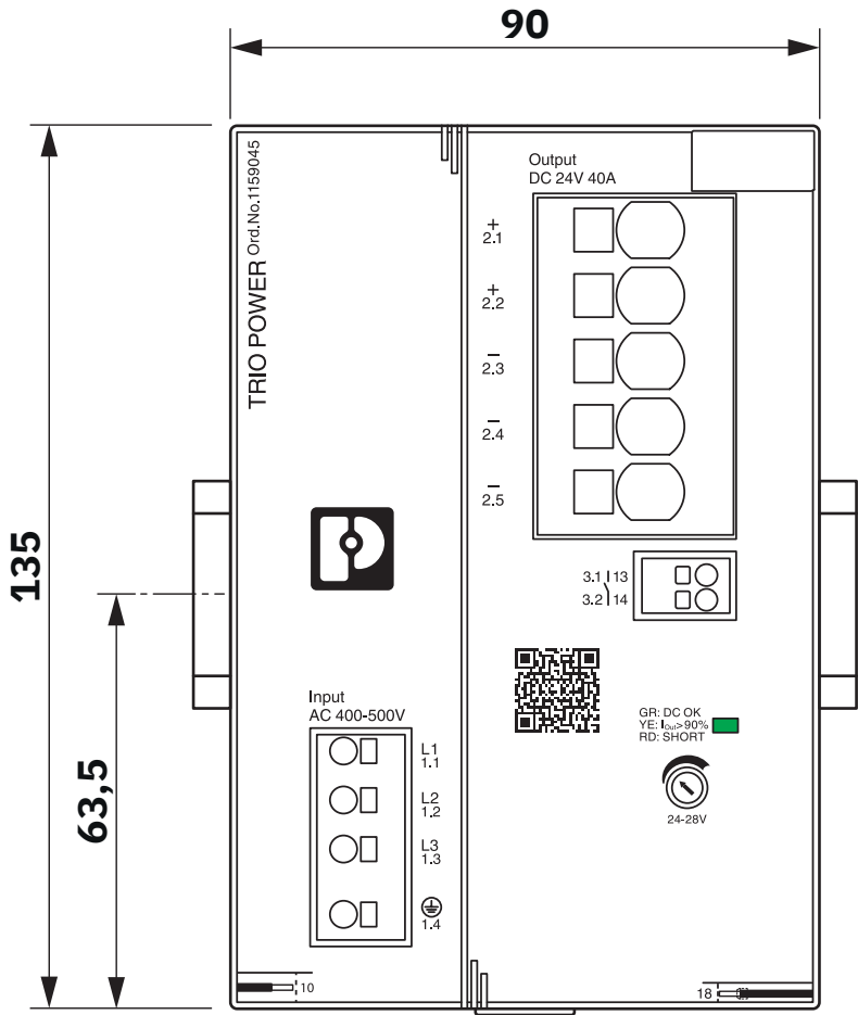
Rysunek wymiarowy
