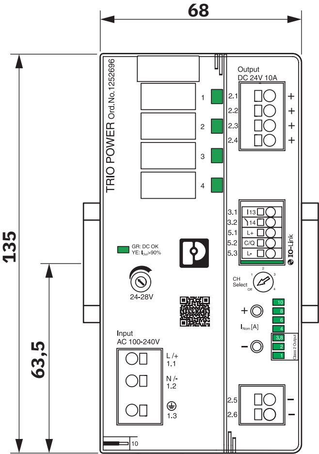
Rysunek wymiarowy
