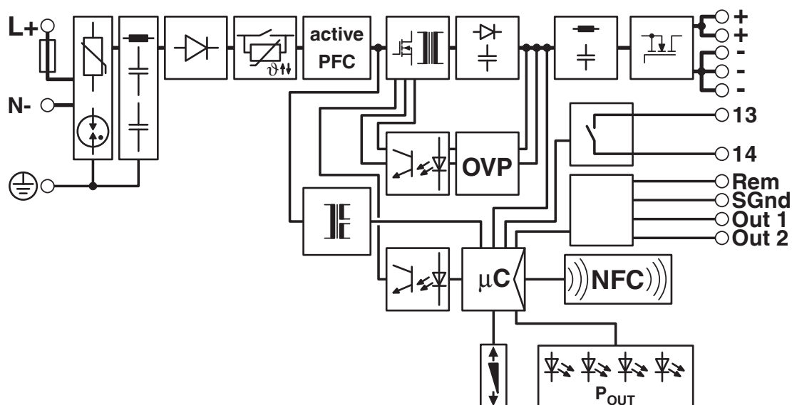
Schemat blokowy
