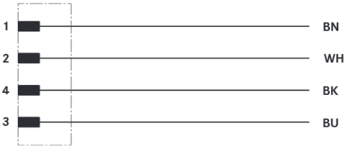
Cable
