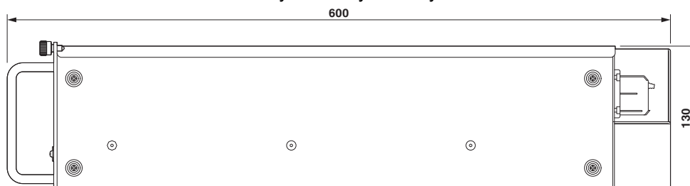
Rysunek wymiarowy
