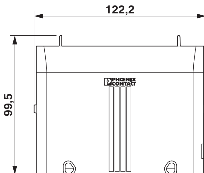
Rysunek wymiarowy
