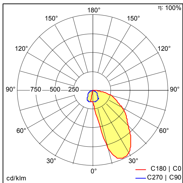
D34983AA_TECTON_C_LED7400-830_L2000_WW_LDE_BK.Idt
