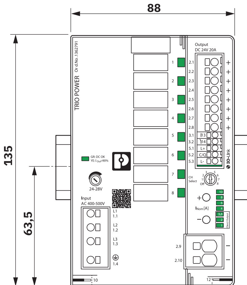
Rysunek wymiarowy
