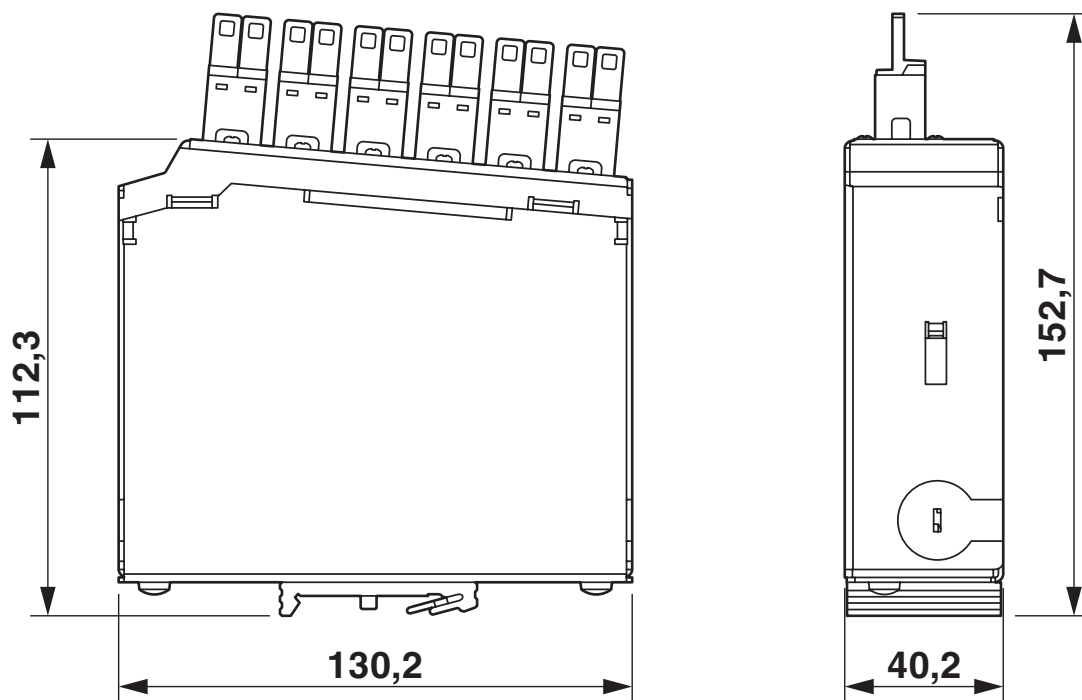
Rysunek wymiarowy
