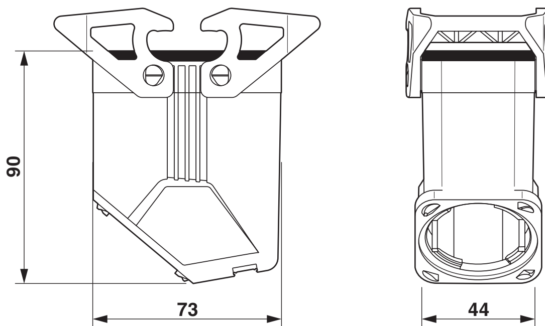
Rysunek wymiarowy
