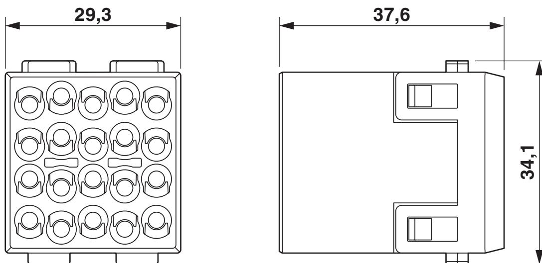
Wkładka styków męskich
