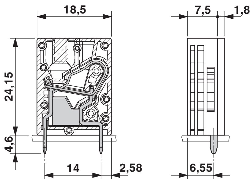
Rysunek wymiarowy
