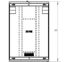
Widok z góry (szerokość 600 mm)
