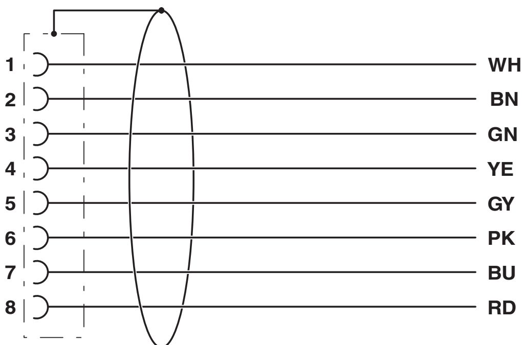
Schemat
