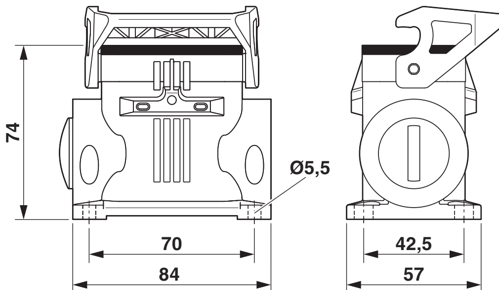
Rysunek wymiarowy
