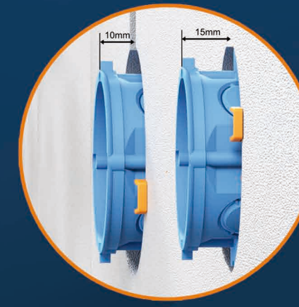
Wybór głębokości osadzenia puszki: 10 mm; 15 mm Zakres: 0 - 20 mm
