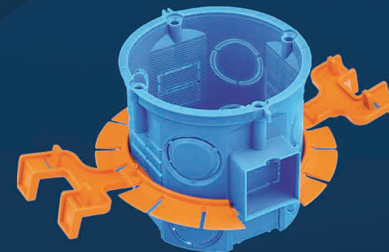
Obcinając diagonalnie łapki wybieramy głębokość osadzenia puszki
