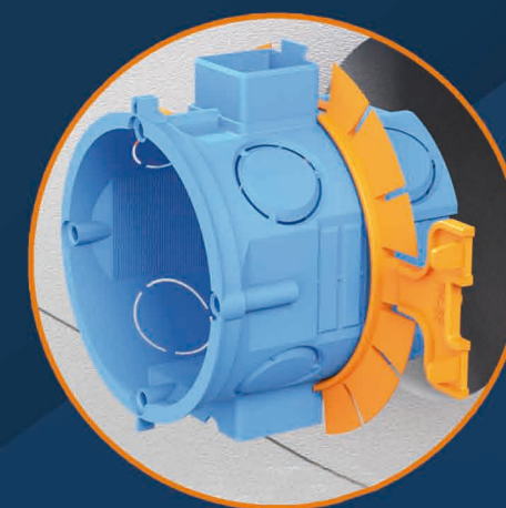
Montaż pierścienia na „klik”
