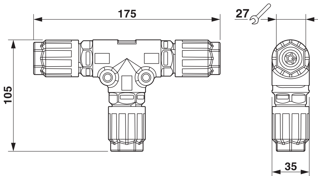
Rysunek wymiarowy
