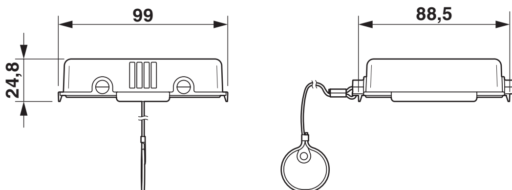
Rysunek wymiarowy
