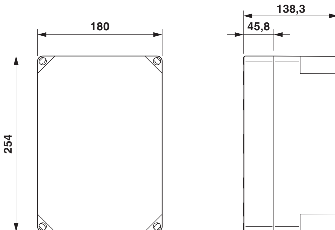
Rysunek wymiarowy
