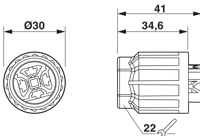
Rysunek wymiarowy
