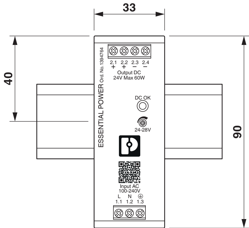
Rysunek wymiarowy
