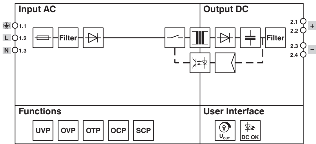
Schemat blokowy
