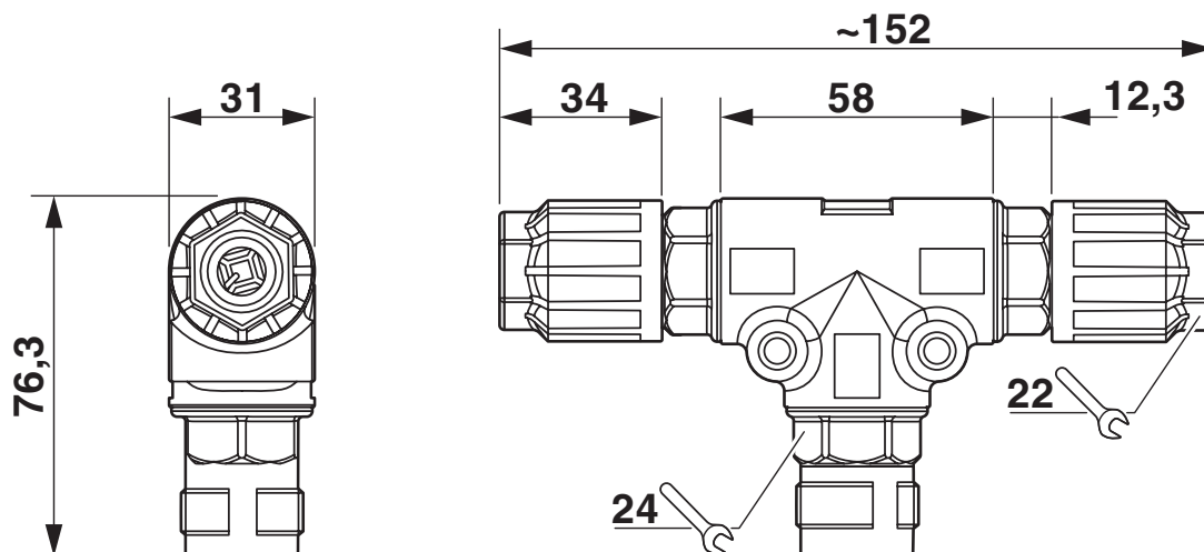
Rysunek wymiarowy
