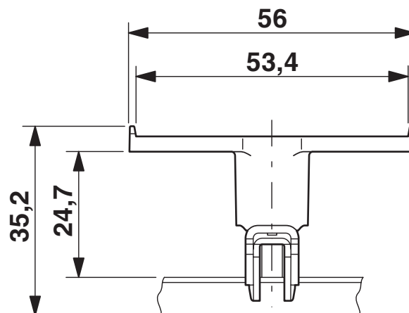
Rysunek wymiarowy
