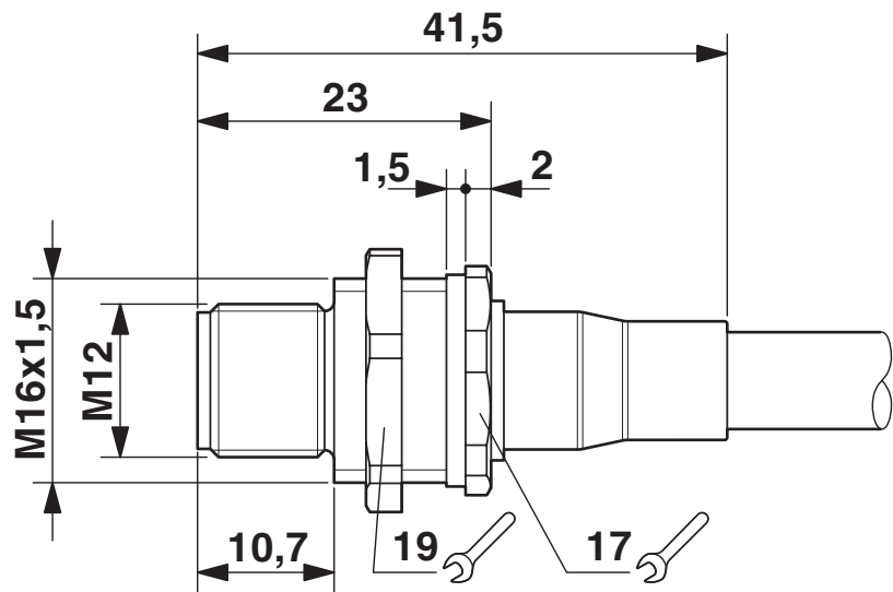
Rysunek wymiarowy
