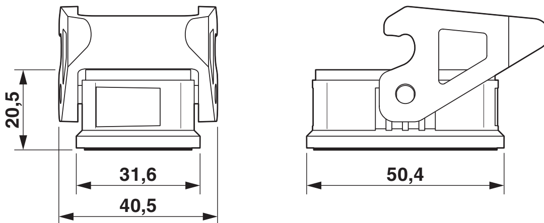
Rysunek wymiarowy
