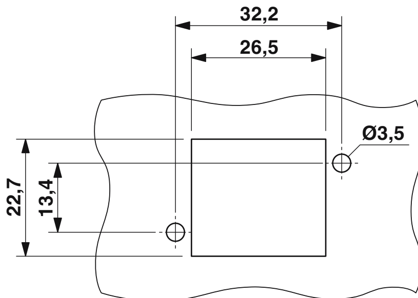
Rysunek wymiarowy
