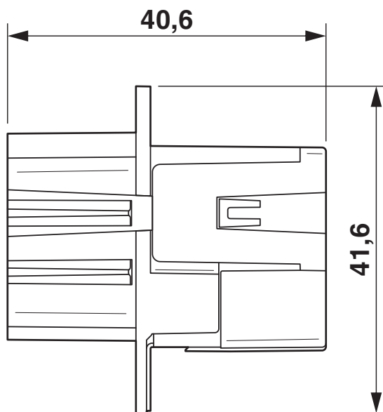
Rysunek wymiarowy
