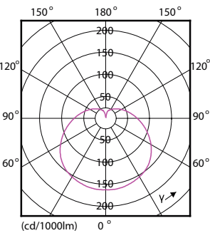
LEDbulb 60W E14 827 FR P48
