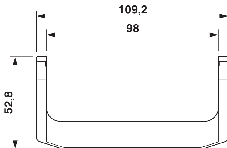
Rysunek wymiarowy
