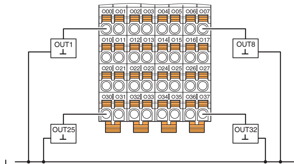
rysunek złączy
