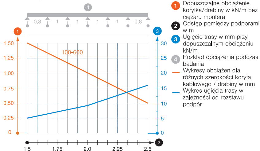
Wykres obciążenia koryta kablowego typ MKS 60
