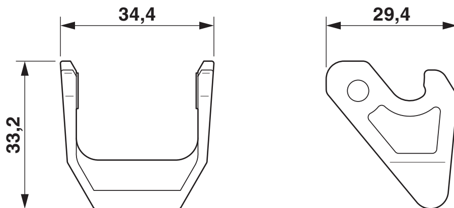
Rysunek wymiarowy
