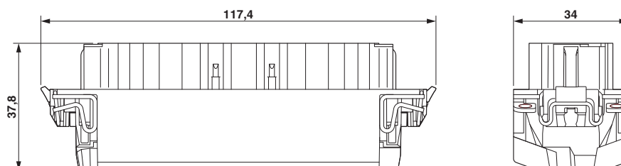
Rysunek wymiarowy
