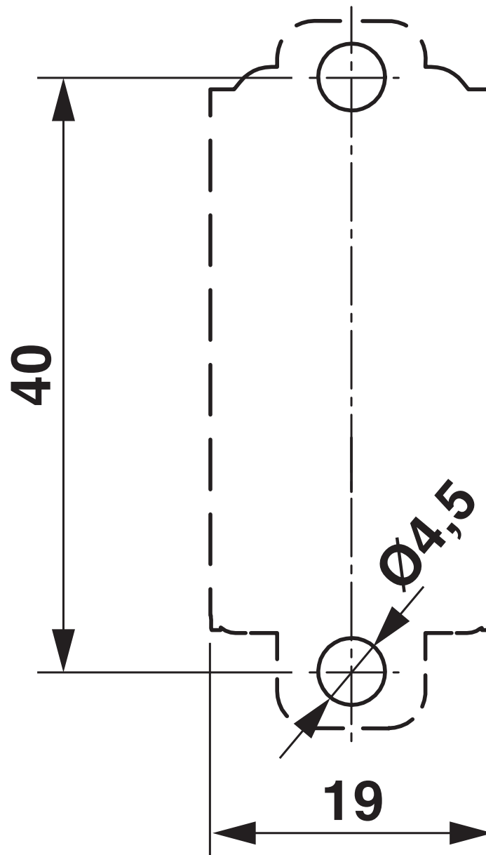
Otworowanie/geometria płytek lutowniczych
