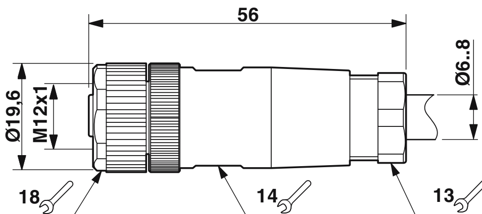
Rysunek wymiarowy
