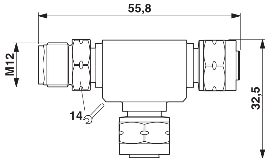
Rysunek wymiarowy
