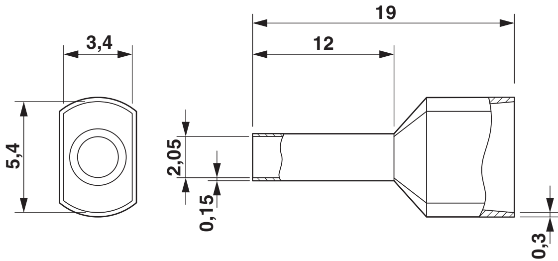
Rysunek wymiarowy
