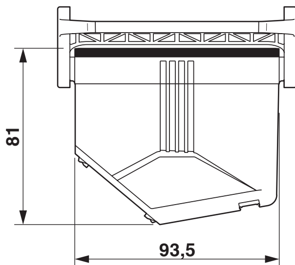
Rysunek wymiarowy
