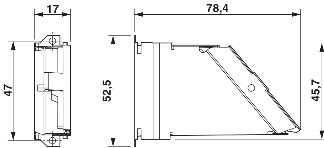
Tuleja wewnętrzna EMC D-SUB
