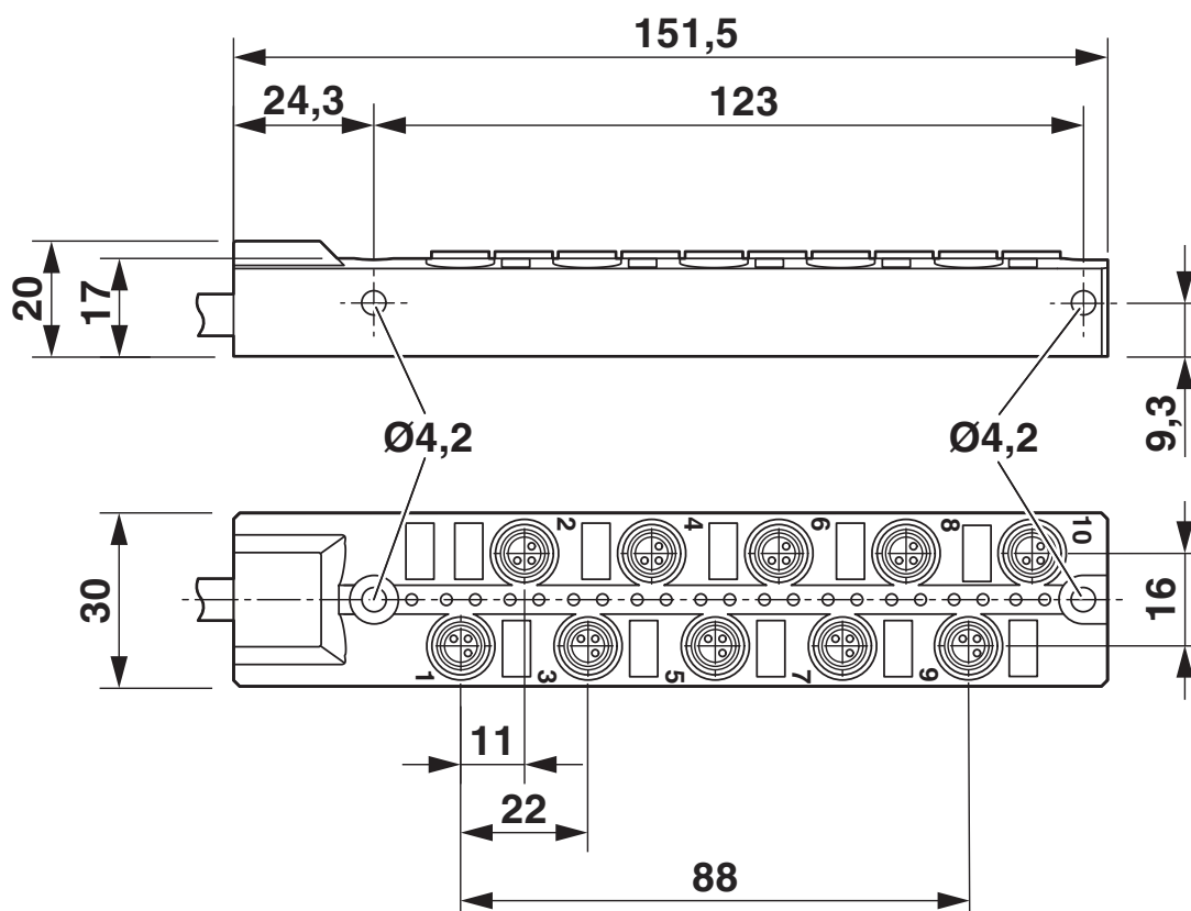
Rysunek wymiarowy
