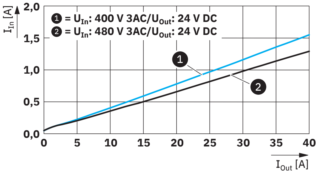
Prąd wejściowy/wyjściowy
