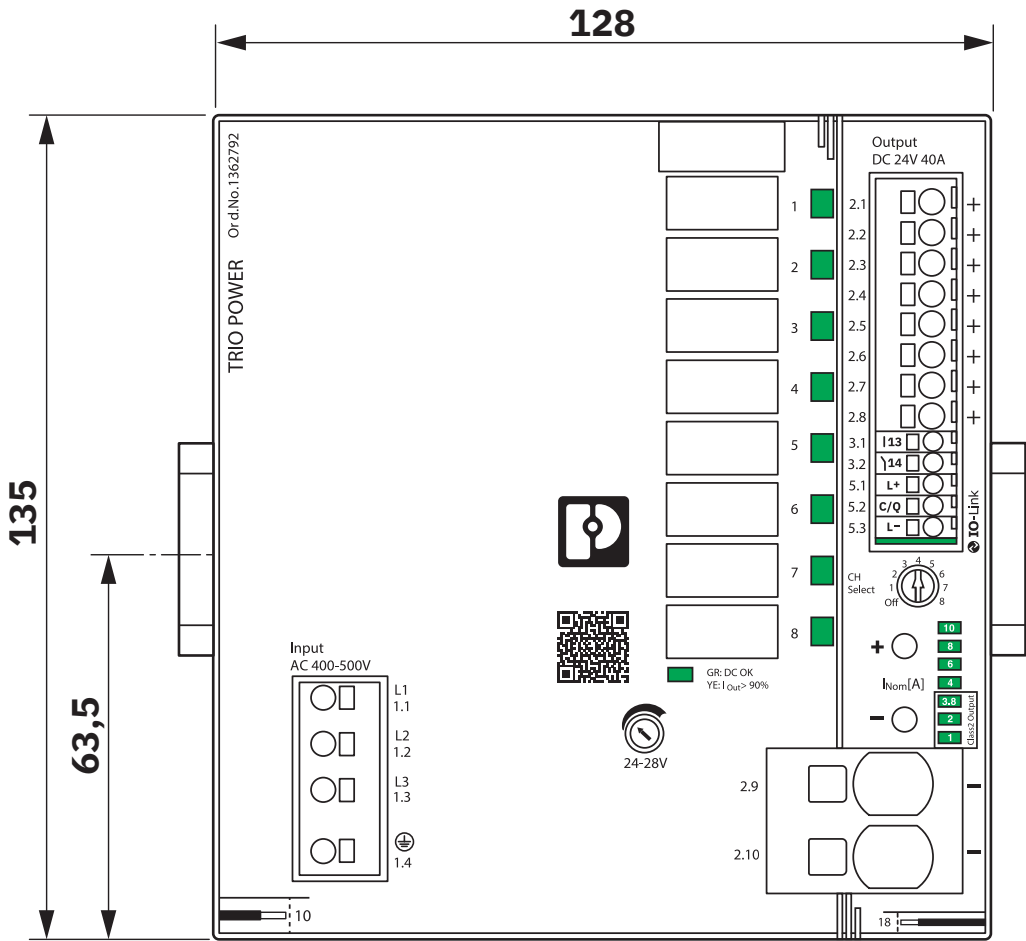
Wymiary urządzenia (wymiary w mm)
