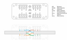
Sekwencja zarabiania modułu połączeniowego WTM08
