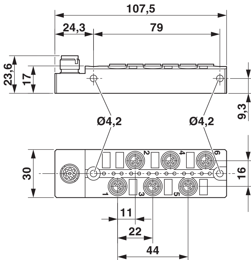
Rysunek wymiarowy
