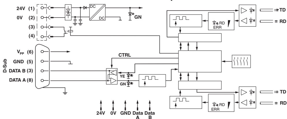
Schemat blokowy
