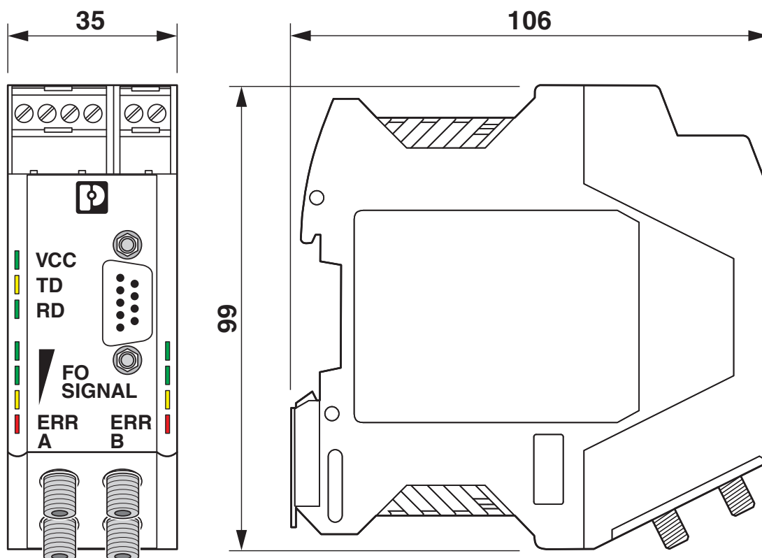
Rysunek wymiarowy
