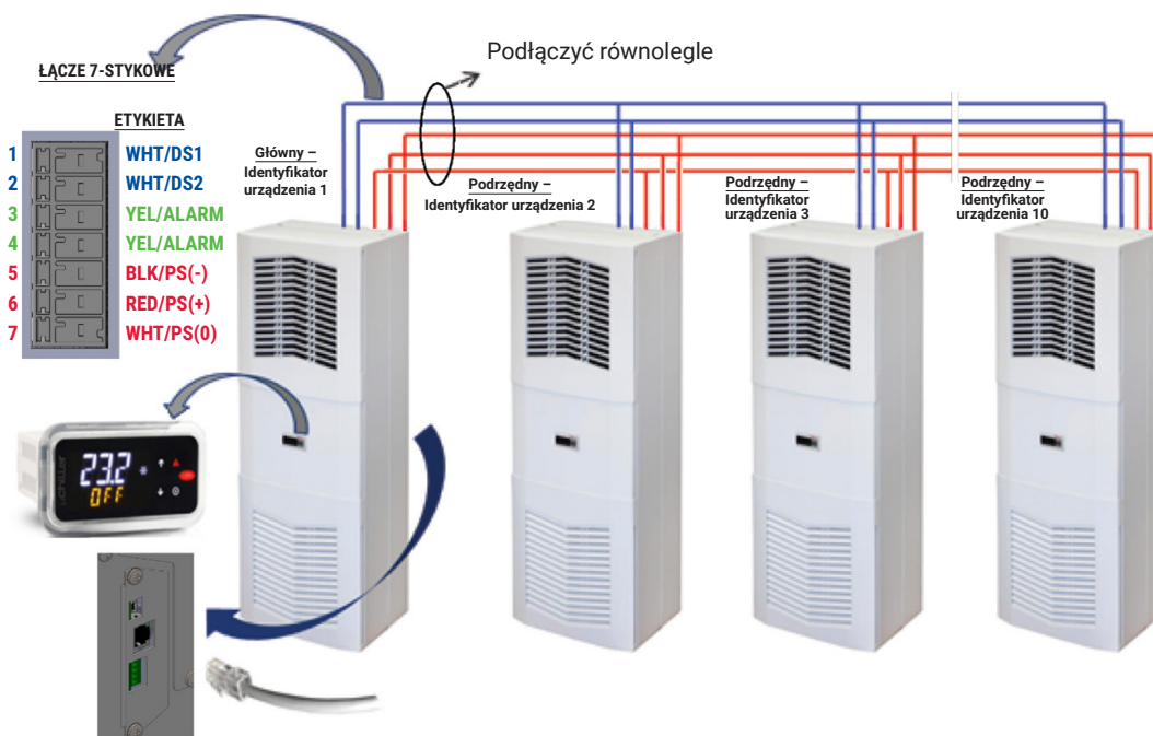
Rysunek 2: Łączność sieciowa w trybie główny–podrzędny
