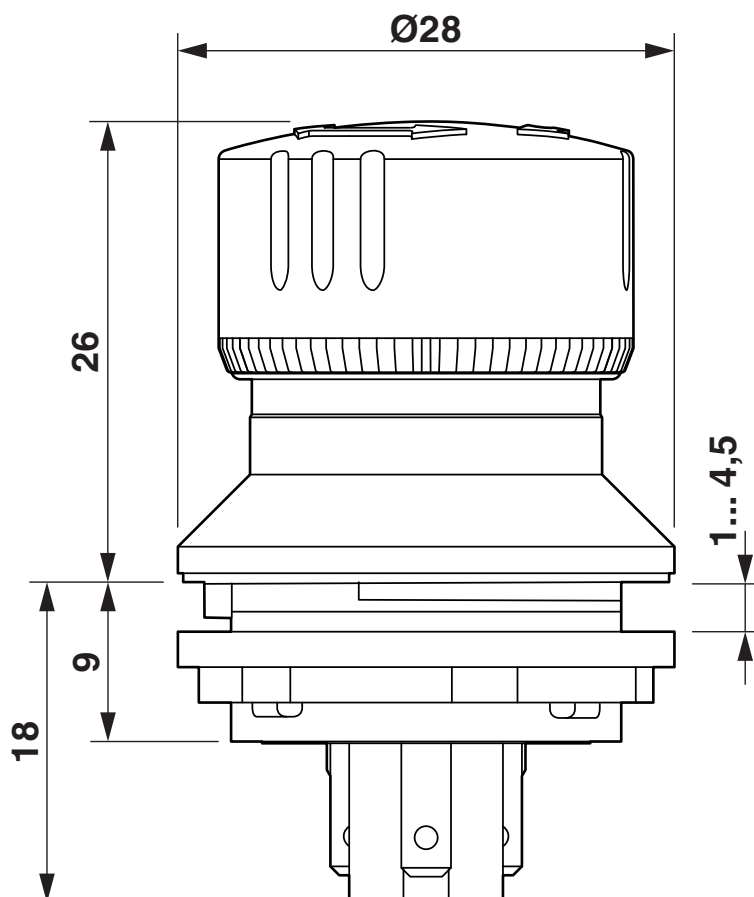
Rysunek wymiarowy
