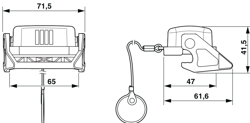
Rysunek wymiarowy
