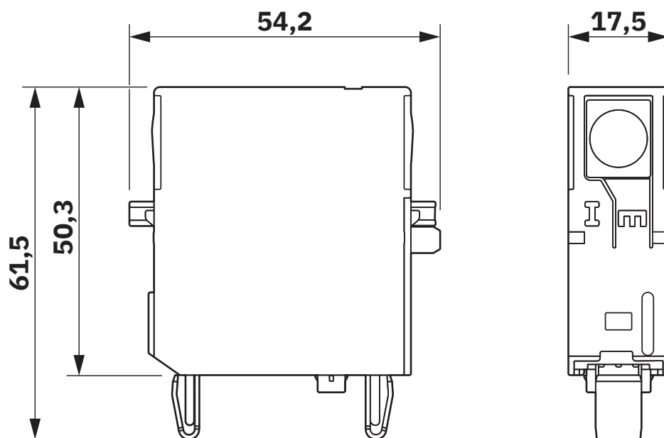
Rysunek wymiarowy
